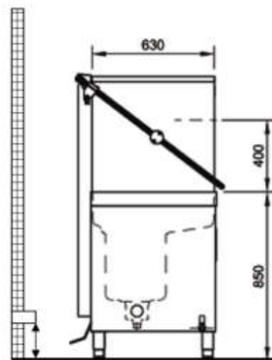
Modell GS 81: Unterkante Ablaufrohr 180 mm
